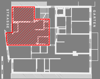
GRUNDRISS
